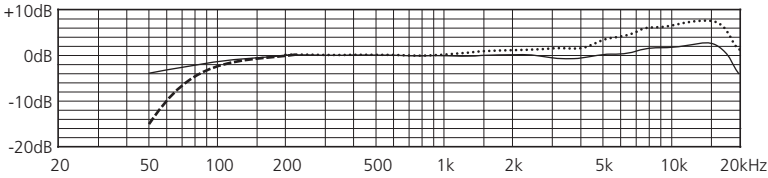
Réponse en fréquence à 0° pour les deux canaux : — sans les filtres - - - avec coupure de basses ..... avec l'augmentation des aigus
