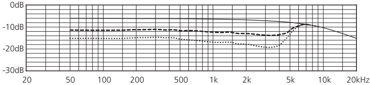
Réponse en fréquence en champ diffus : — avec le transducteur avant seul (CMIT) - - - SuperCMIT, Preset 1 ..... SuperCMIT, Preset 2
