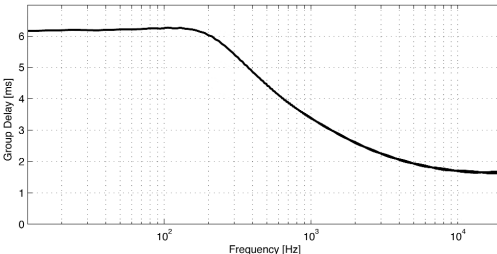
Canal 1: latence en fonction de la fréquence
